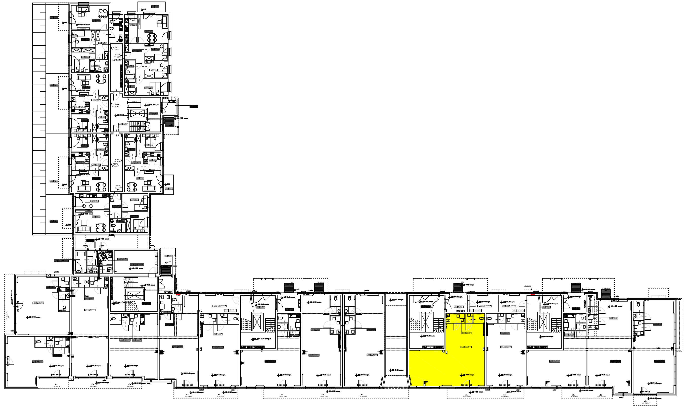
BUDYNEK B1 RZUT PARTERU
