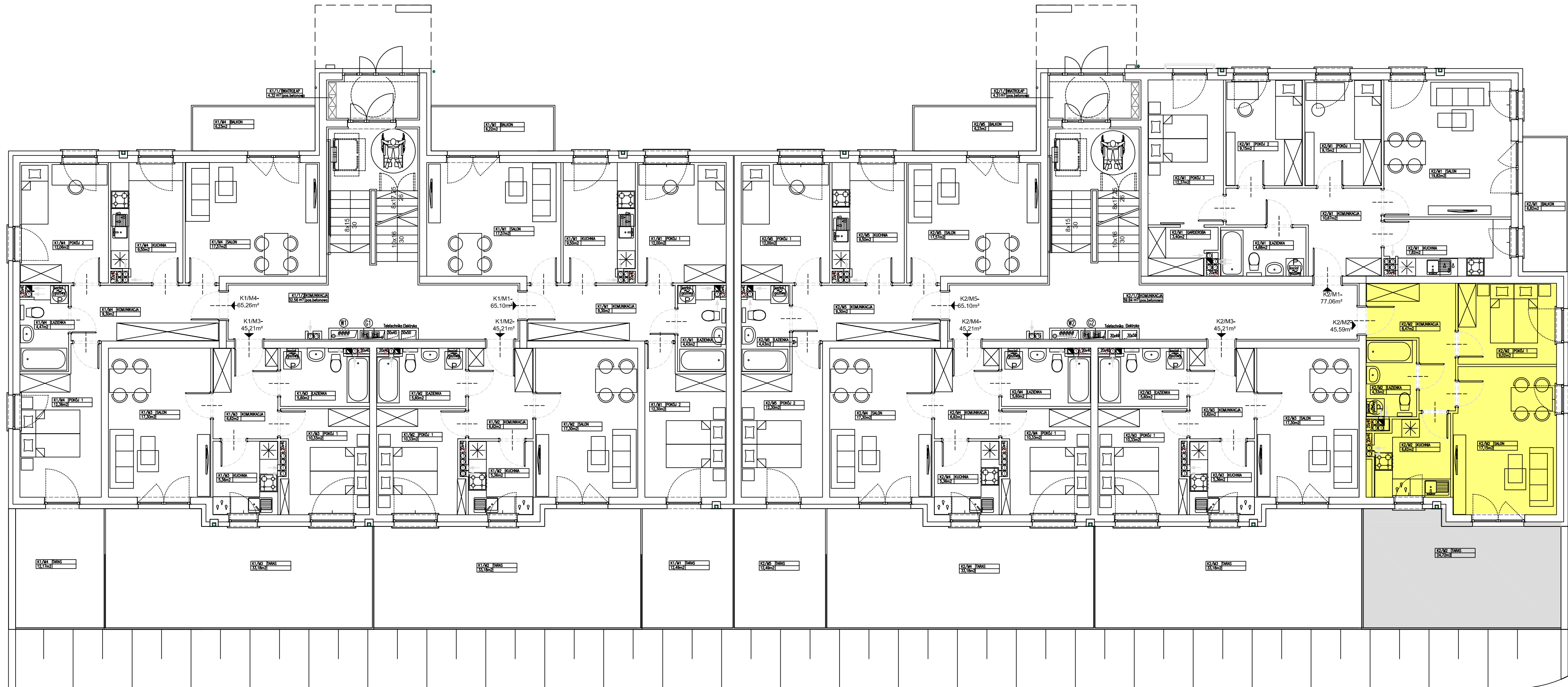
LEŚMIANA IV - BUDYNEK B2 RZUT PARTERU
